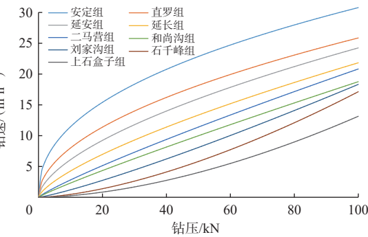
图 5 各层位钻速与钻压的关系
