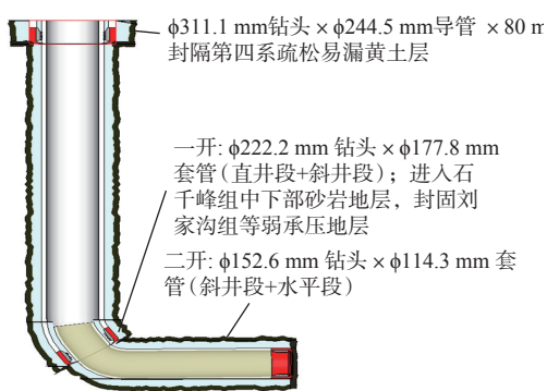
图2 新二开水平井井身结构
