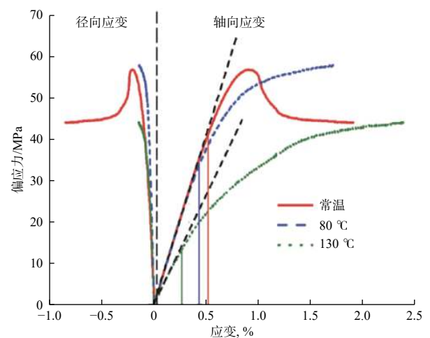
图2 高温循环载荷下的水泥石偏应力-应变曲线 [17]
