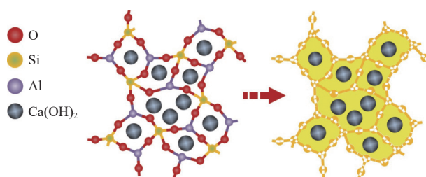
图 3 防腐水泥浆体系设计思路
