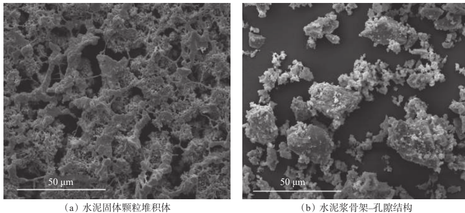
图1 典型水泥浆“液-固”态转化期的典型微观结构
