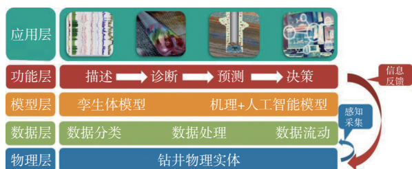
图 4 钻井数字孪生系统整体架构示意
