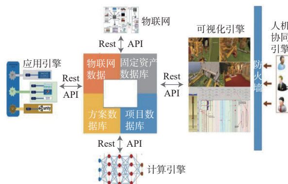
图6 钻井数字孪生系统中驱动引擎的分块构建
